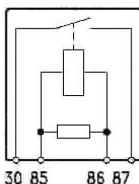
Рисунок 31 – Схема расположения контактов реле
