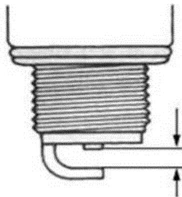
Рисунок 28 - Зазор между электродами свечи зажигания
