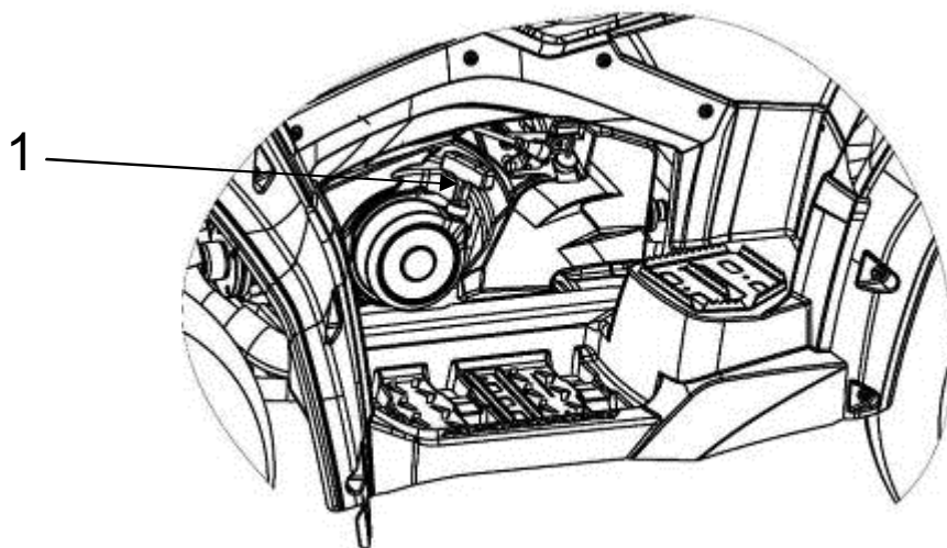
1 – Ручка ручного стартера
