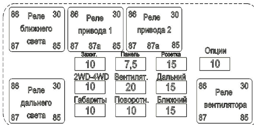
Рисунок 30 – Блок предохранителей и реле
